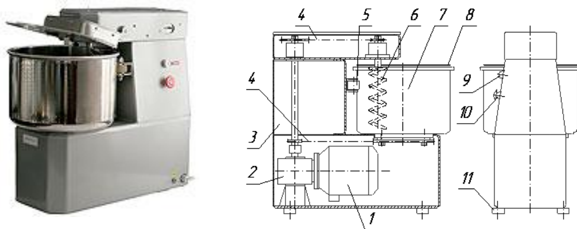
Рисунок 1. Тестомесильная машина МТ-12
