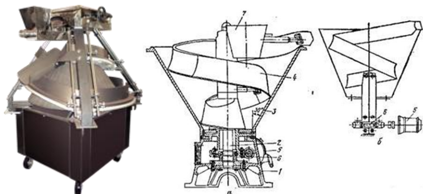
Рисунок 3. Округлитель ХТО-2500
