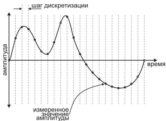
Рис.1 Процесс дискретизации
