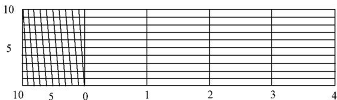
Рисунок 1 – Поперечный масштаб
