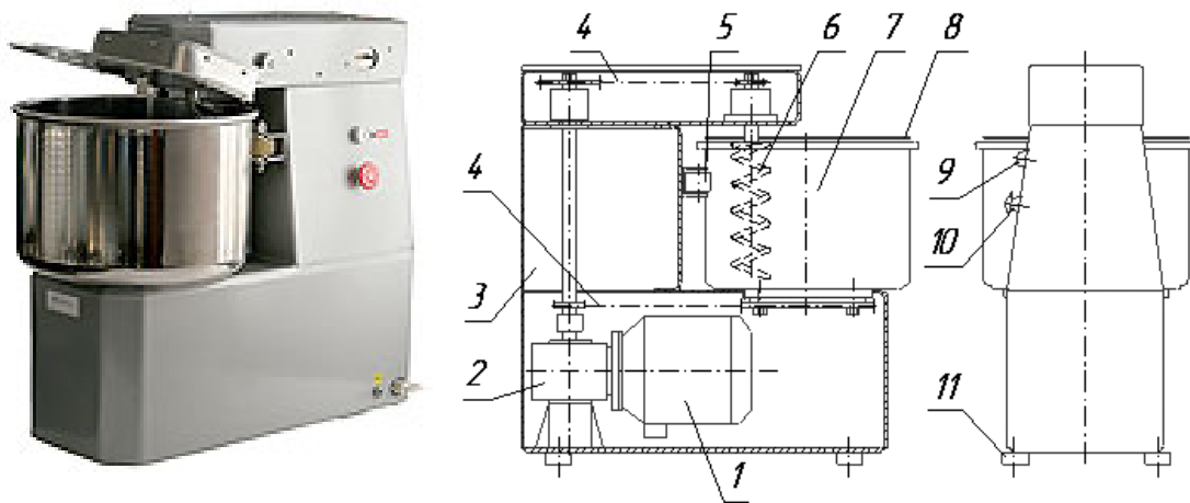
Рисунок 1. Тестомесильная машина МТ-12
