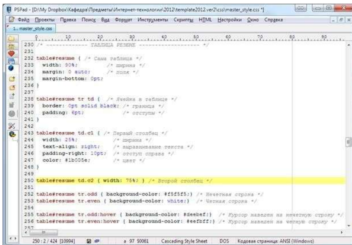
Рис. 13 – Описание идентификатора #resume во внешняя таблица стилей master_style.css в среде редактора PSPad
