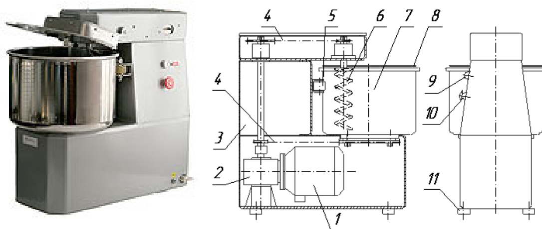
Рисунок 1. Тестомесильная машина МТ-12
