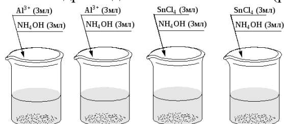
Рис. 16. Порядок проведения опыта: а – г – пробирки с соответствующими растворами. В пробирки вводить растворы Al^{3+} (5%-ный) и SnCl_4 (30%-ный) по каплям до полного растворения осадков.
