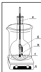
Рис. 19. Схема исполнения опыта: а - термометр для определения первой капли дифениламина(ДФА)- начальной температуры плавления( t_{\text{нач}} ) и конечной температуры ( t_{\text{кон}} )- по плавлению всей массы ДФА в капилляре; б- капилляр с ДФА; в- столбик ДФА; г-водяная баня; д -
