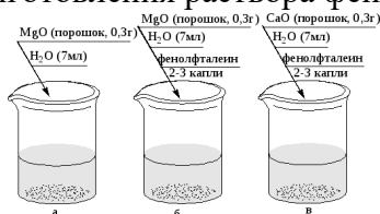
Рис. 14. Порядок проведения опыта: а, б – пробирки с оксидом магния; в – пробирка с оксидом кальция.
