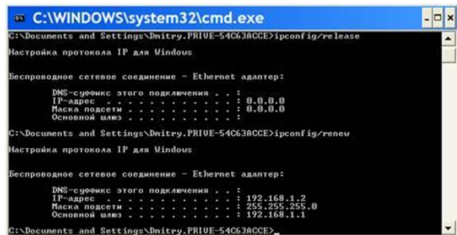
Рис. 16 - Обновление данных соединения при помощи командной строки
