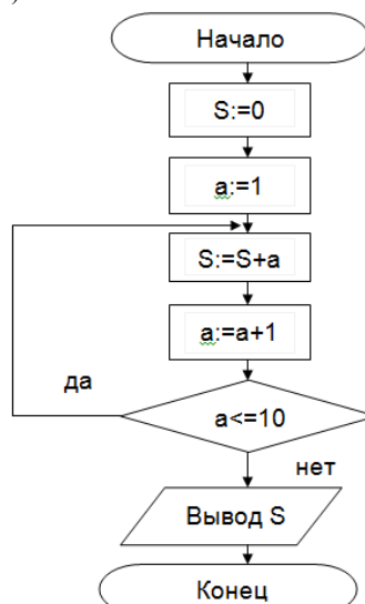
Рисунок 4. Циклический алгоритм с постусловием
