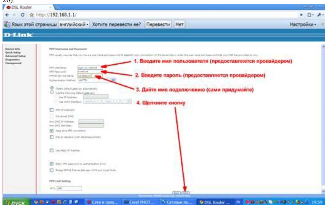
Рис. 20 - Ввод данных для авторизации
