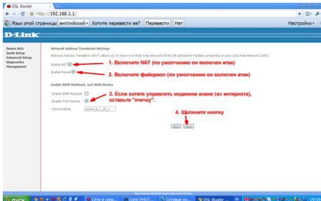
Рис. 21 - Включение NAT и фаервола
