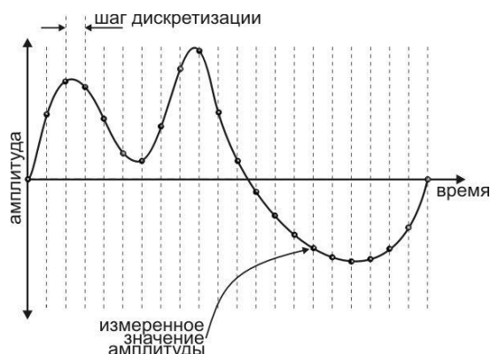
Рис.1 Процесс дискретизации
